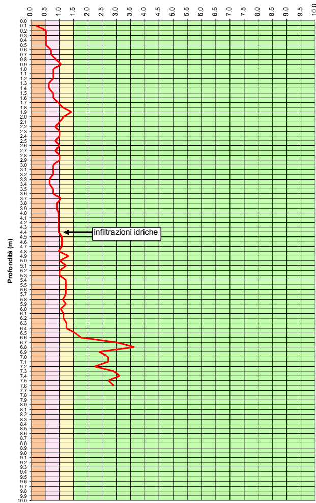
PROVA PENETROMETRICA P14
