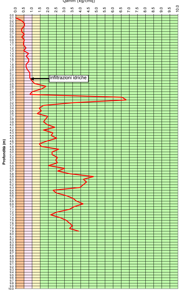
PROVA PENETROMETRICA P13
