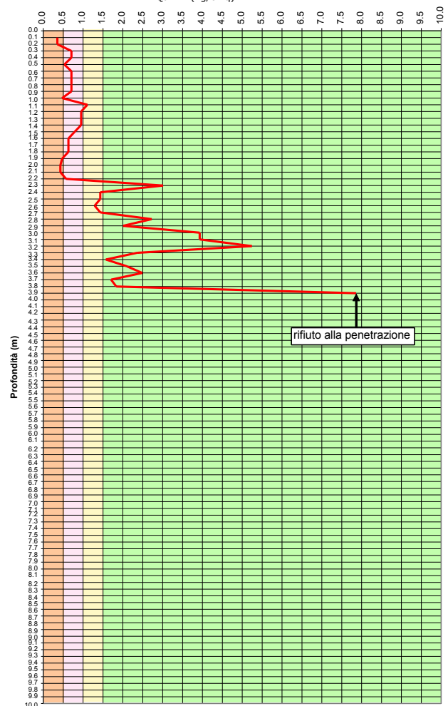
PROVA PENETROMETRICA P8
