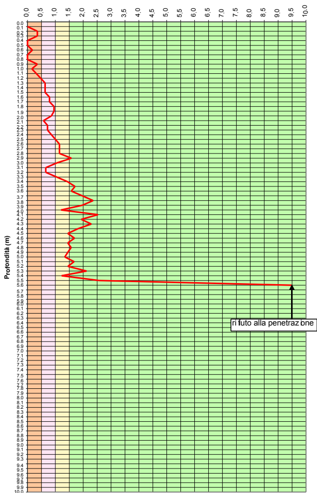
PROVA PENETROMETRICA P9
